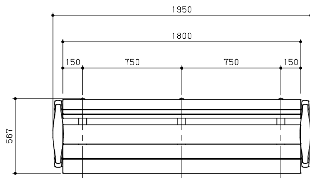
平面図 S = 1 / 20
