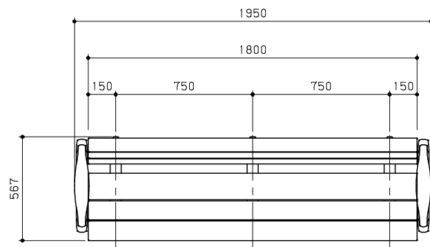
平面図 S = 1 / 20
