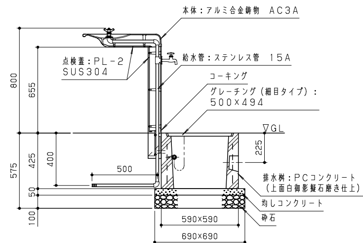
断面図 S = 1 / 20
