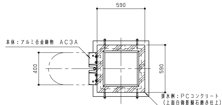
排水枳伏図 S = 1 / 20
