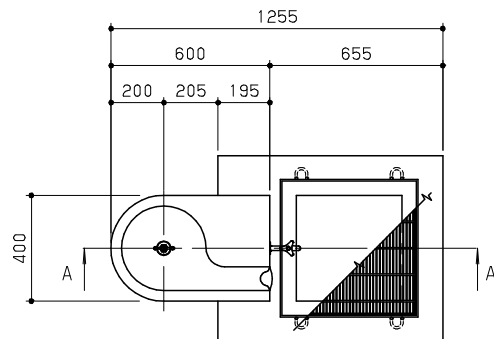
平面図 S=1/20
