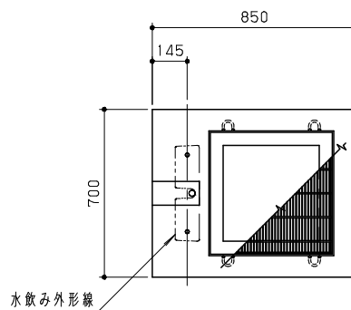
配置図 S=1/20
