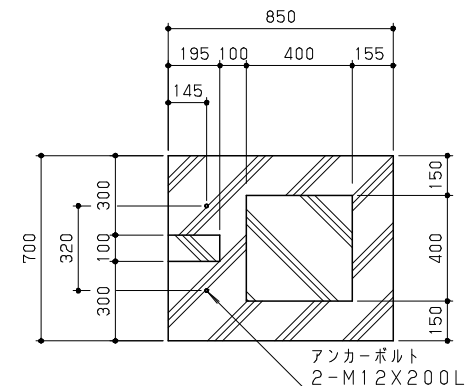
B-B断面図 S=1/20
