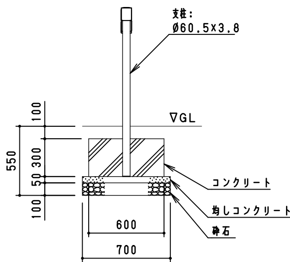
側面図 S=1/30
