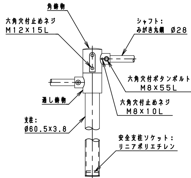
鋳物部／柱脚部詳細図 S=1/10
