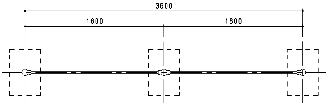
平面図 S=1/30
