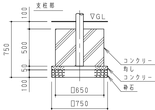
基礎詳細図 S = 1 / 30
