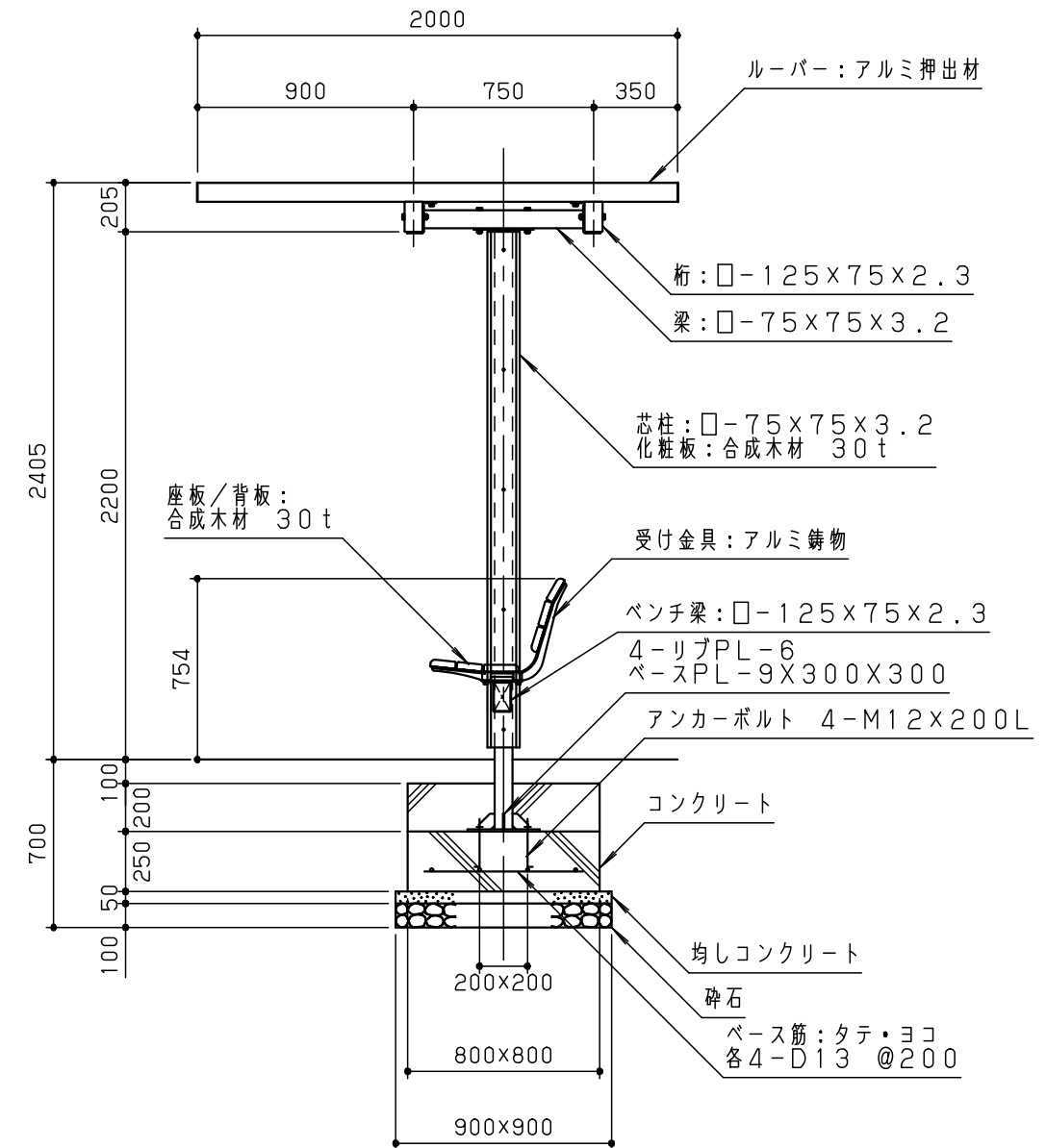
断面図 S = 1 / 30
