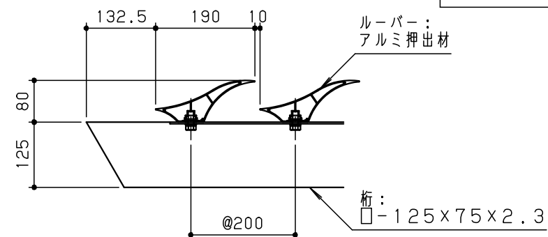
栈木断面図 S = 1 / 10
