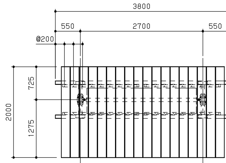
平面図 S = 1 / 50
