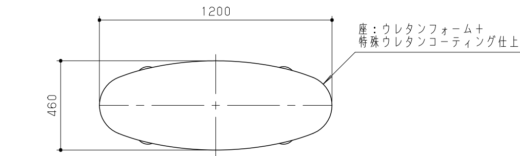
平面図 S = 1 / 20
