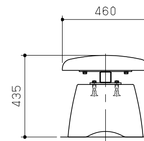
側面図 S = 1 / 20
