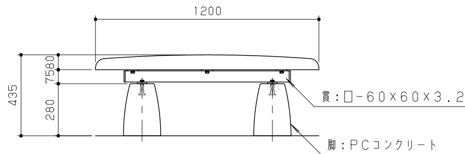
立面図 S = 1 / 20
