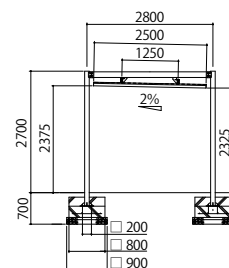
PAS-A2 ¥1,760,000 (税抜) 6390 W × 2800 D × 2700 H ・ 615kg
