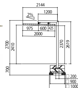
PAS-B2 ¥1,410,000 (税抜) 6390 W × 2144 D × 2700 H ・ 435kg
