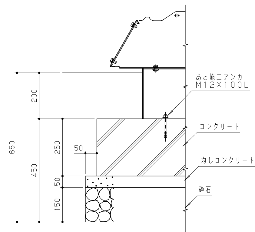
基礎断面図 S = 1 / 10
