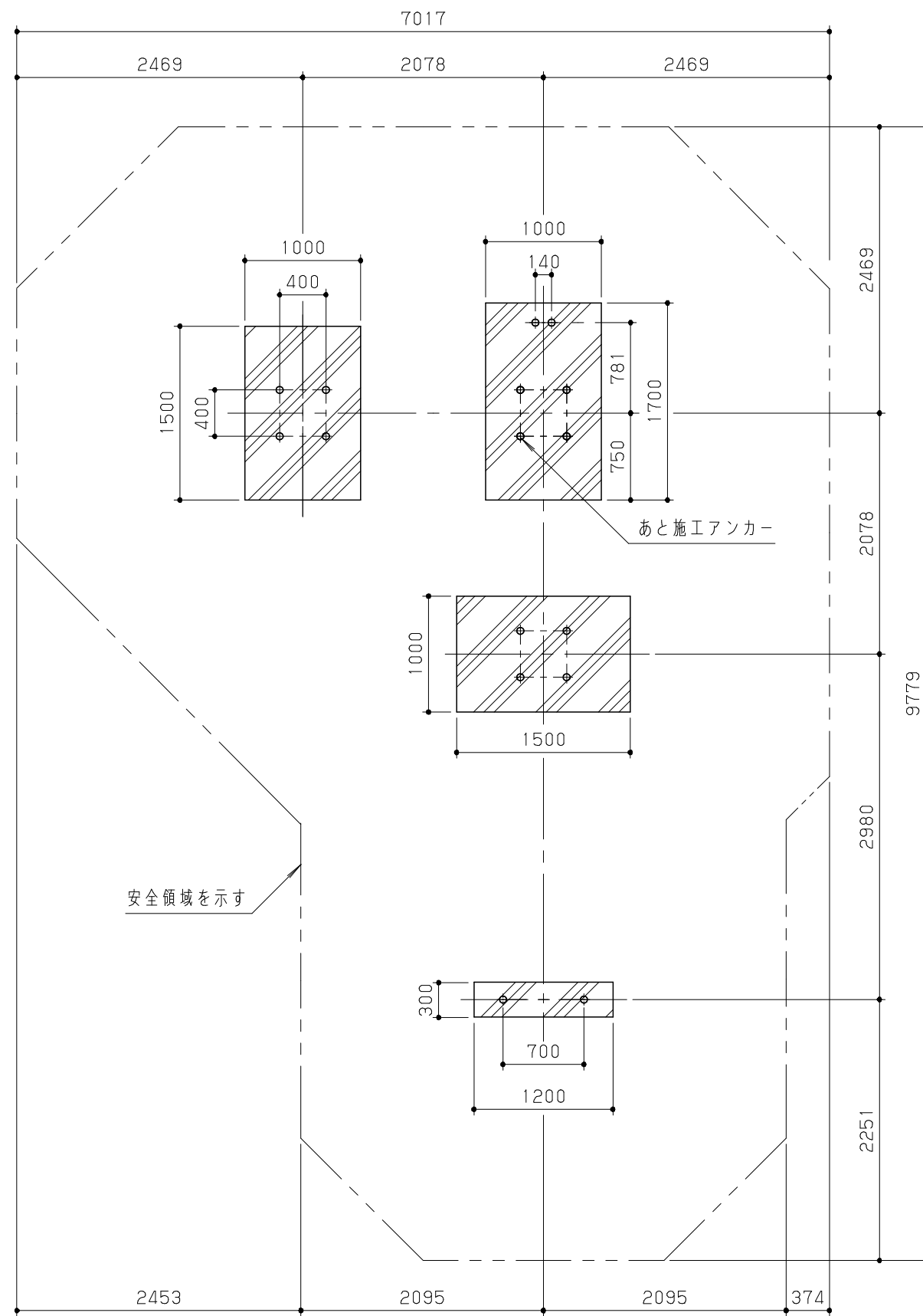
基礎伏図 S = 1 / 50
