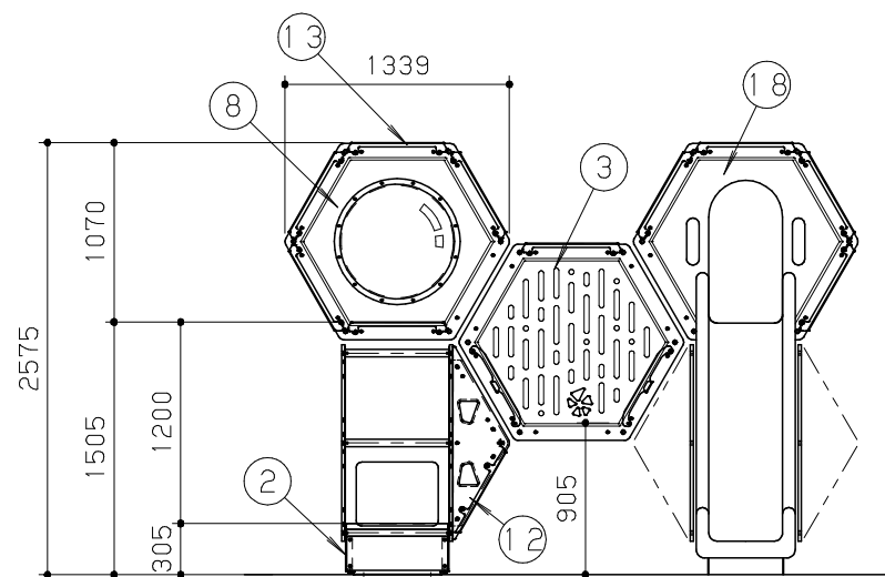
A 視 立 面 図 S = 1 / 5 0
