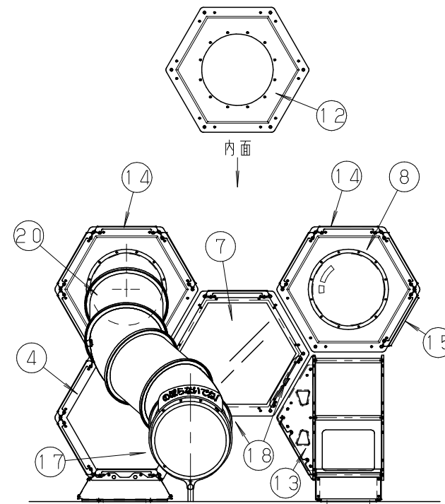
D 視
