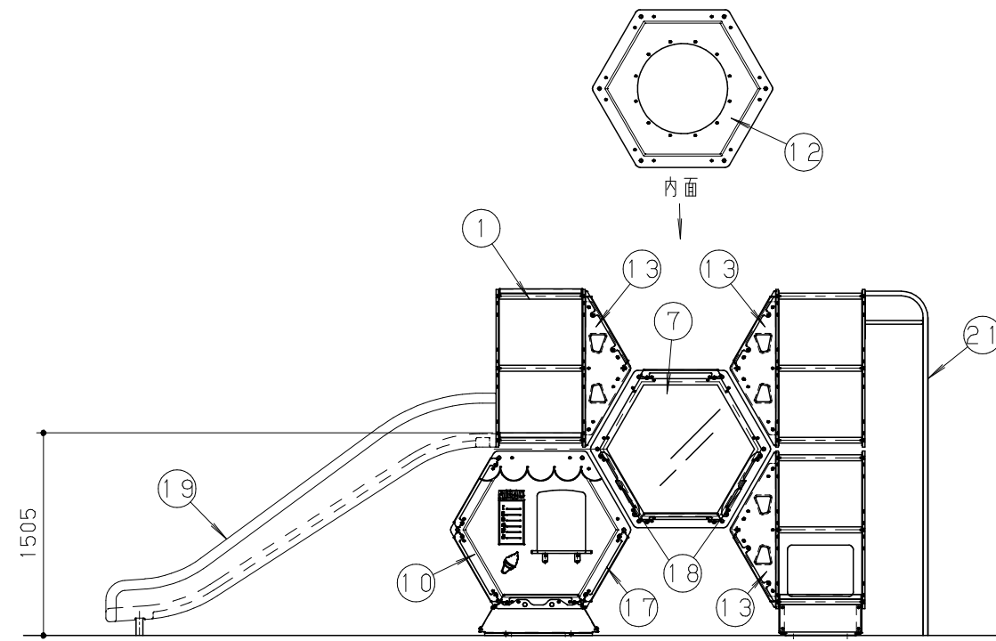
B 視
