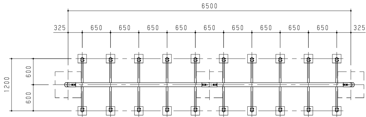
立面図 S = 1 / 50
