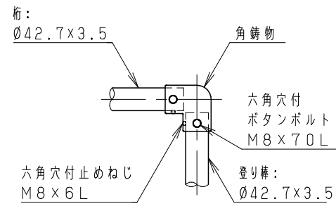
B 詳細図 S = 1 / 10
