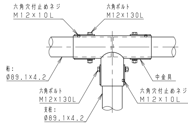
C 詳細図 S = 1 / 10
