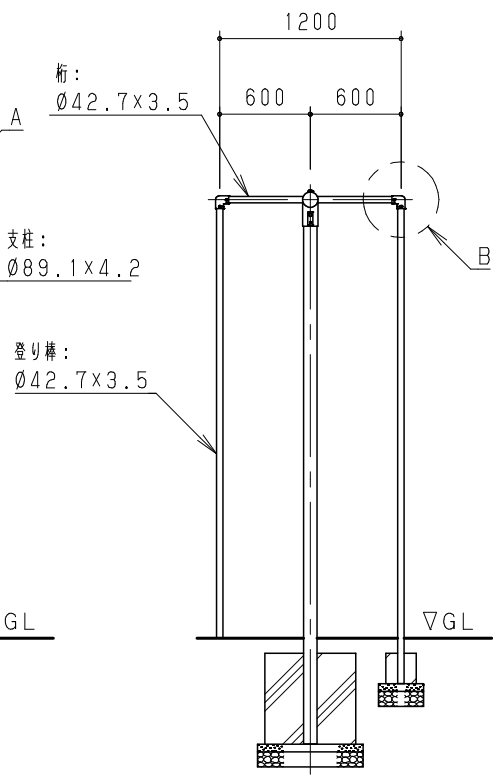
側面図 S = 1 / 50
