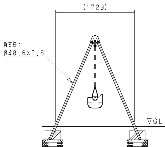
側面図 S = 1 / 50
