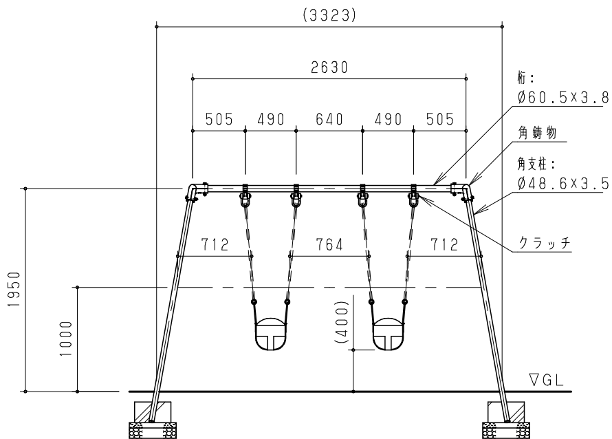
立面図 S = 1 / 50
