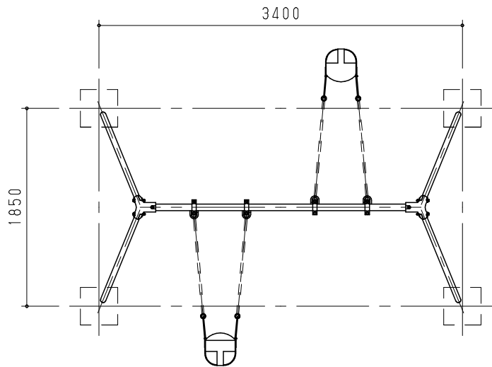
平面図 S = 1 / 50
