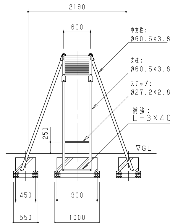
側面図 S = 1 / 50
