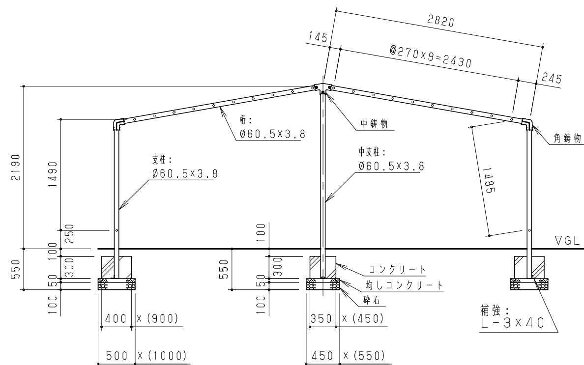
立面图 S = 1/50
