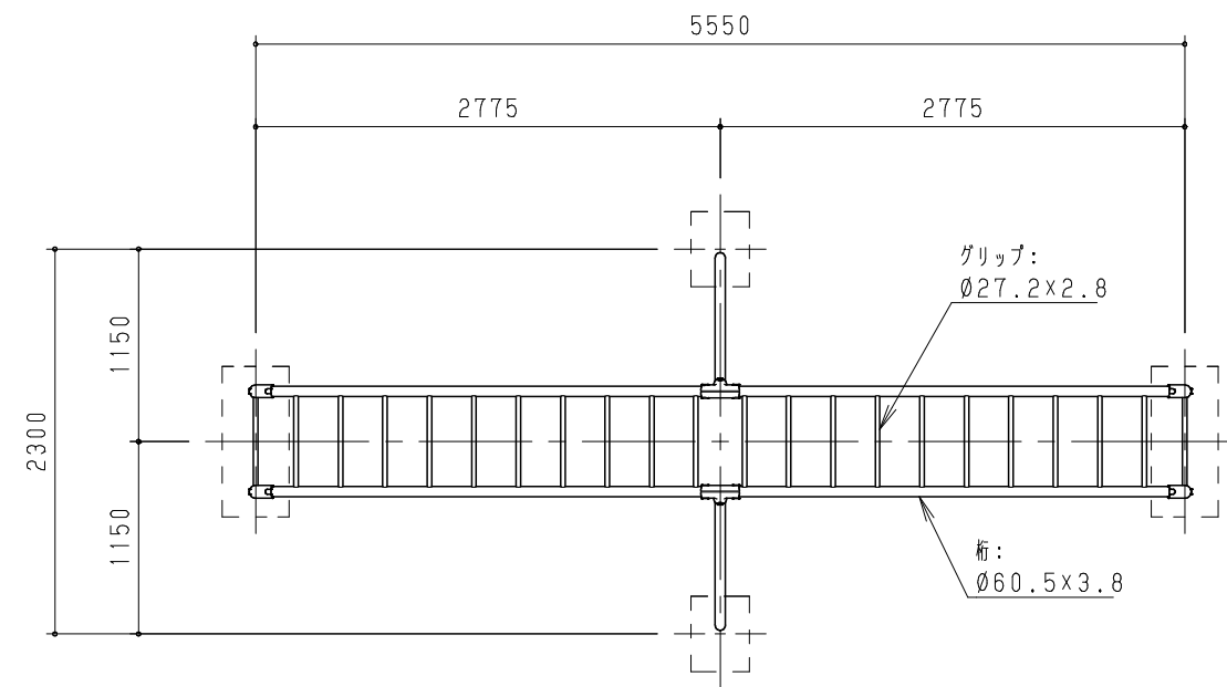
平面図 S = 1 / 50
