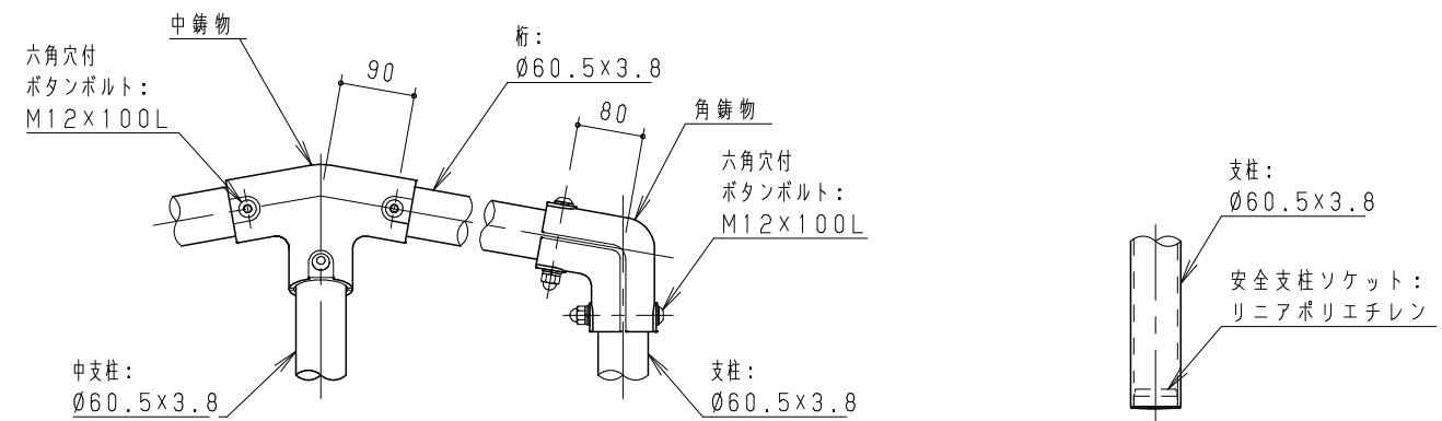
鑄物部詳細図 S = 1 / 10
