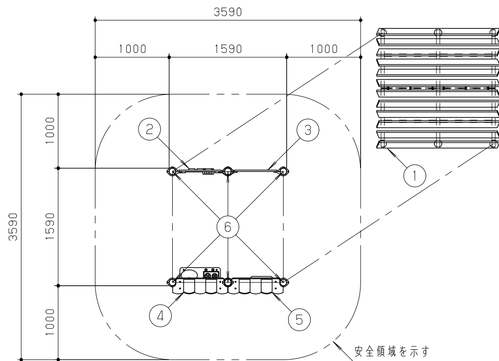
平面図 S = 1 / 50
