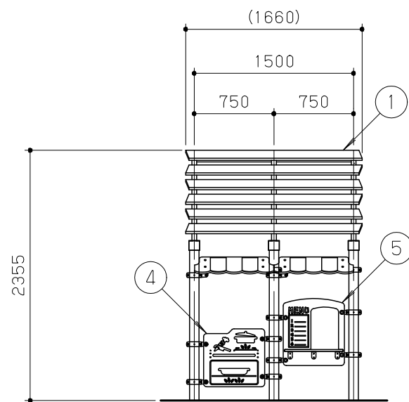
立面図 S = 1 / 50
