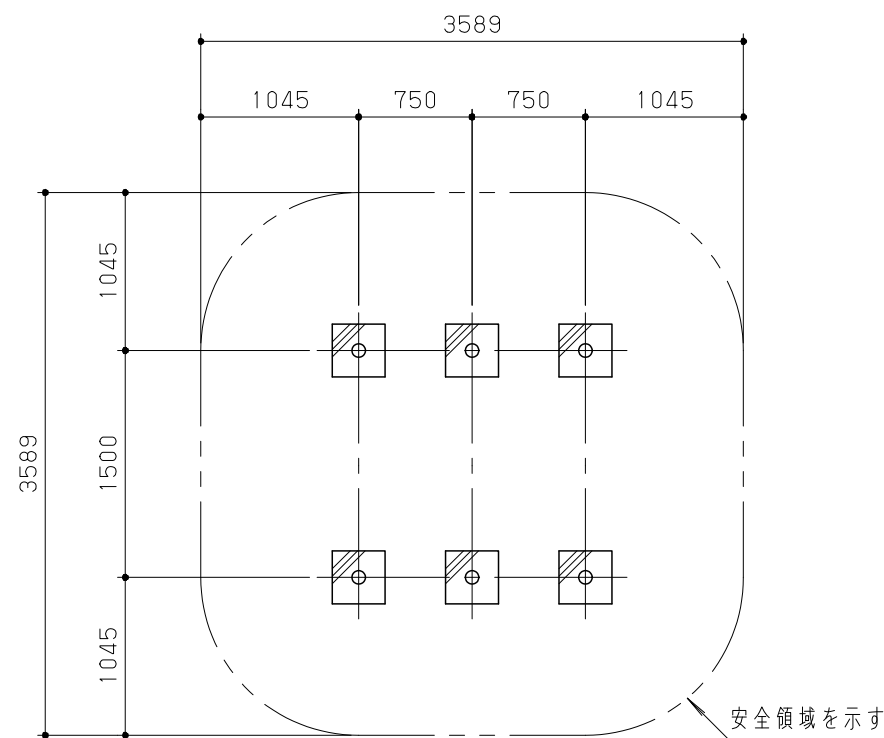
基礎伏図 S = 1 / 50
