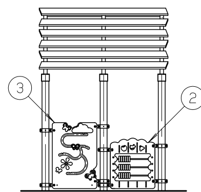
立面図 S = 1 / 50
