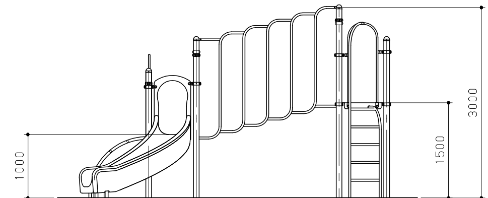
B 視 立 面 図 S = 1 / 6 0
