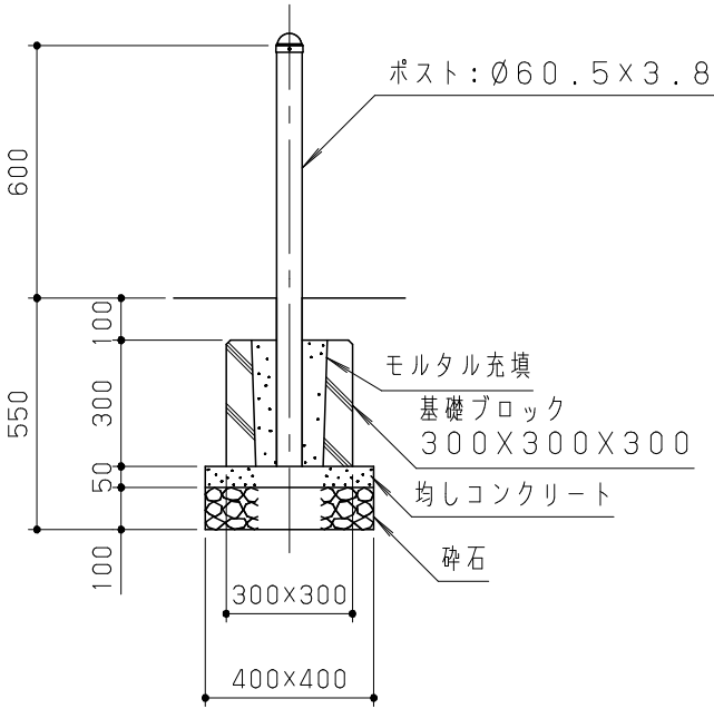
側面図 S = 1 / 20
