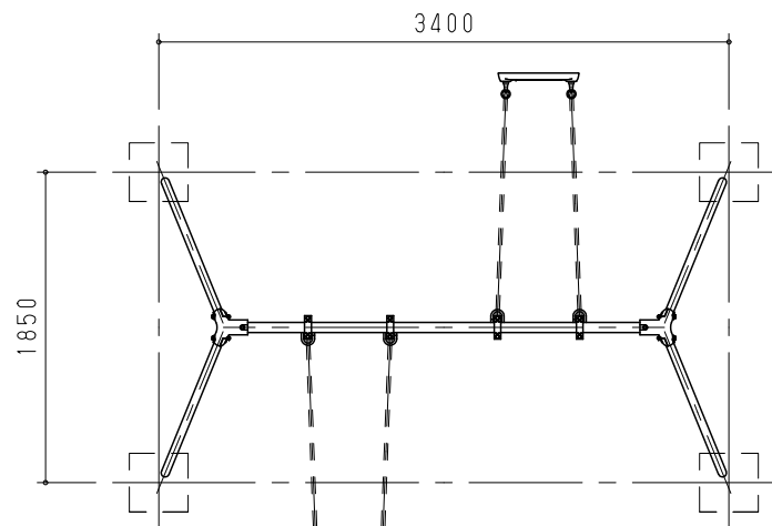
平面図 S = 1 / 50
