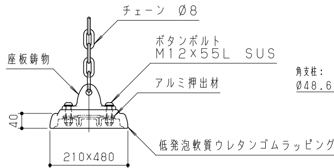
座板詳細図 S = 1 / 10
