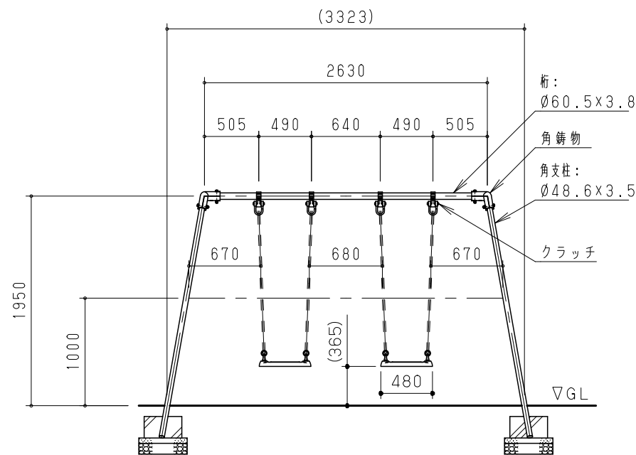
立面図 S = 1 / 50
