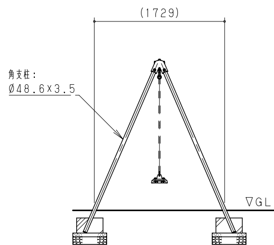
側面図 S = 1 / 50
