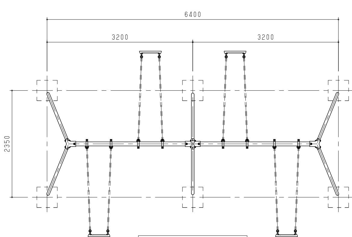
平面図 S = 1 / 50
