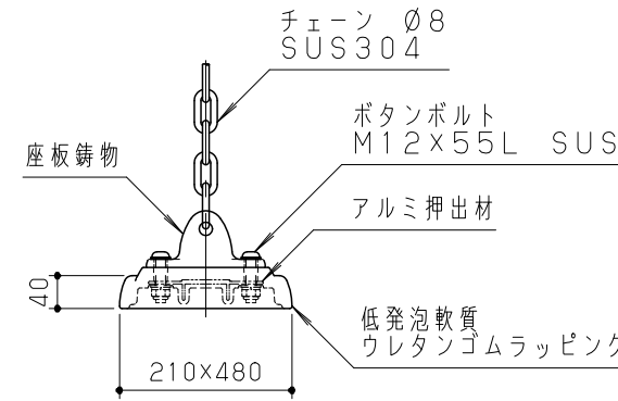
座板詳細図 S = 1 / 10
