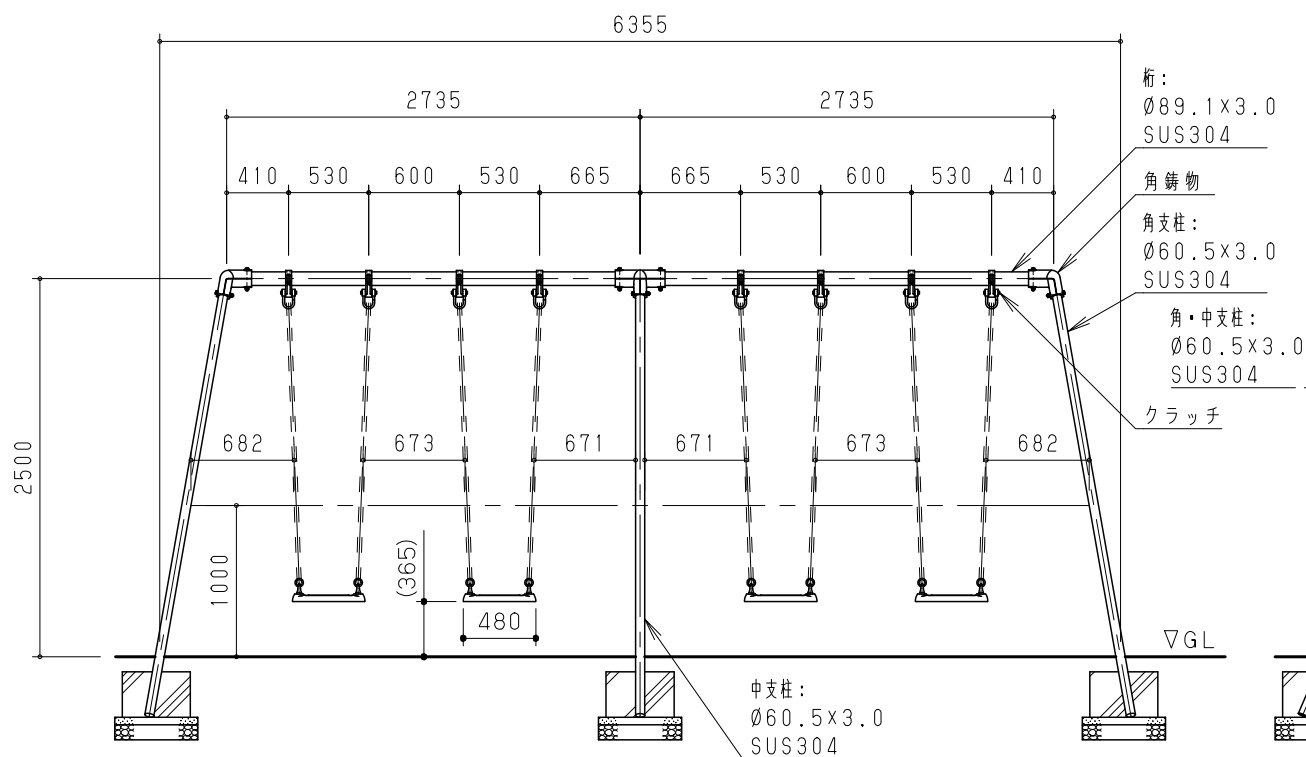
立面図 S = 1 / 50
