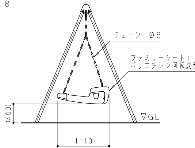
側面図1 S = 1 / 50
