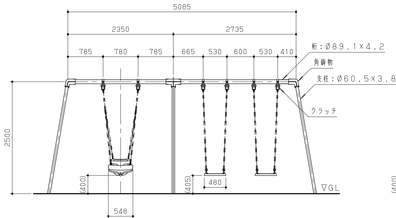
立面図 S = 1 / 50
