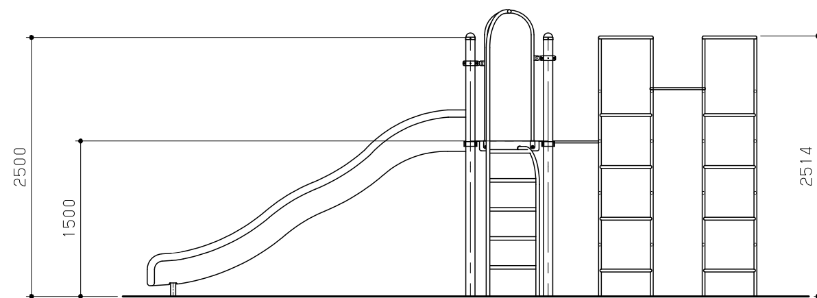
C 視立面図 S = 1 / 50
