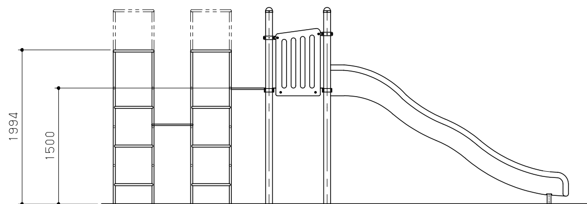
A 視立面図 S = 1 / 50
