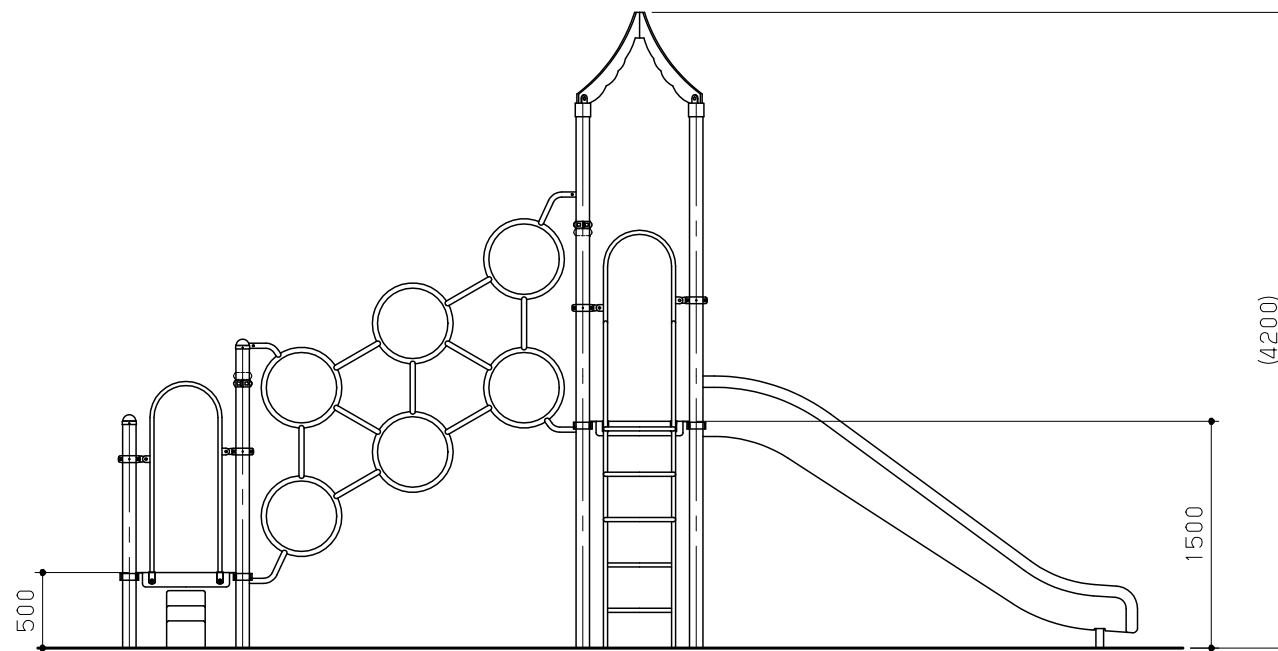
A 視 立 面 図 S = 1 / 5 0
