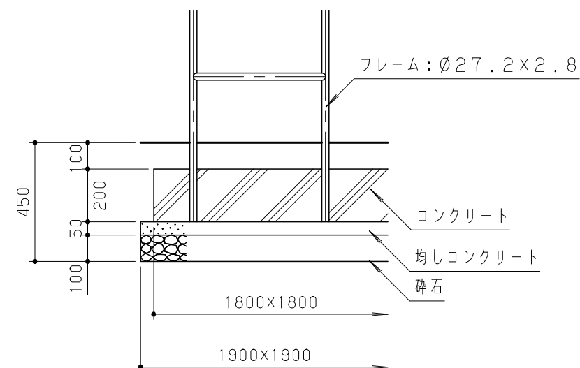
基礎F1断面詳細図 S = 1 / 20
