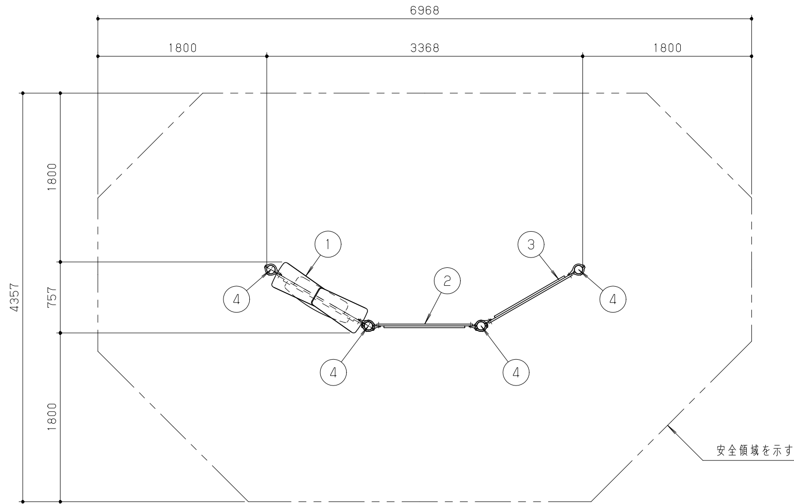
平面図 S = 1 / 40
