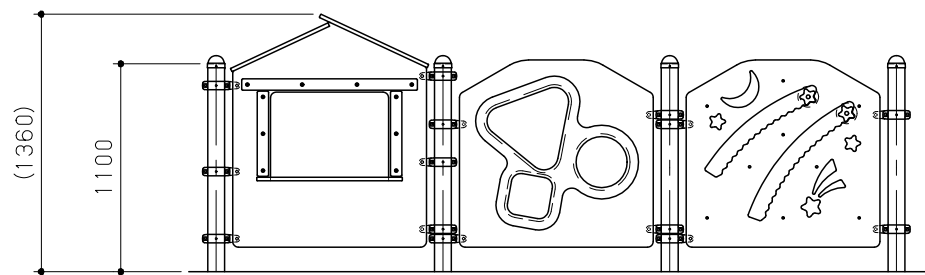
展開図 S = 1 / 40
