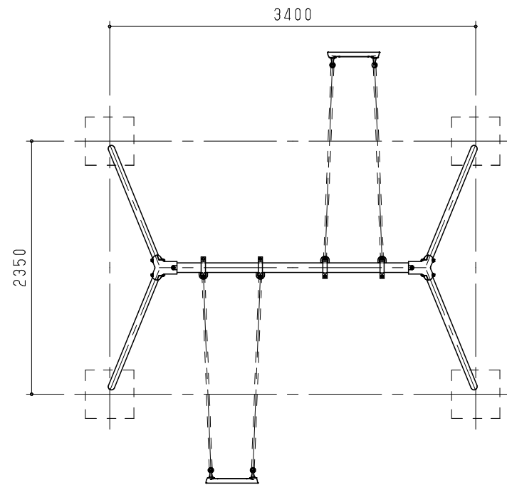
平面図 S = 1 / 50
