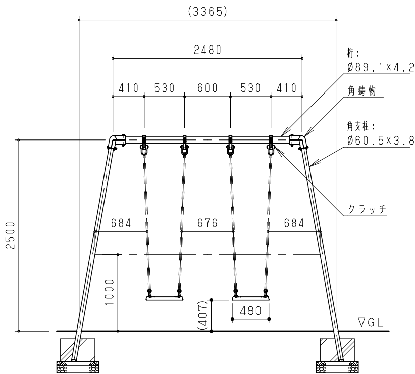
立面図 S = 1 / 50
