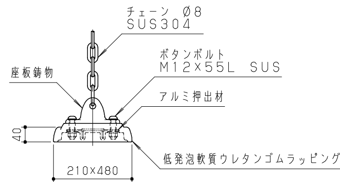
座板詳細図 S = 1 / 10
