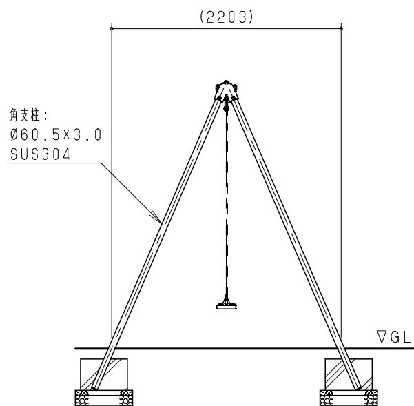
側面図 S = 1 / 50
