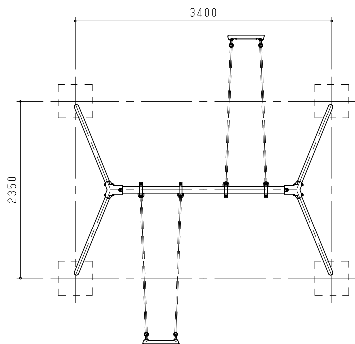
平面図 S = 1 / 50
