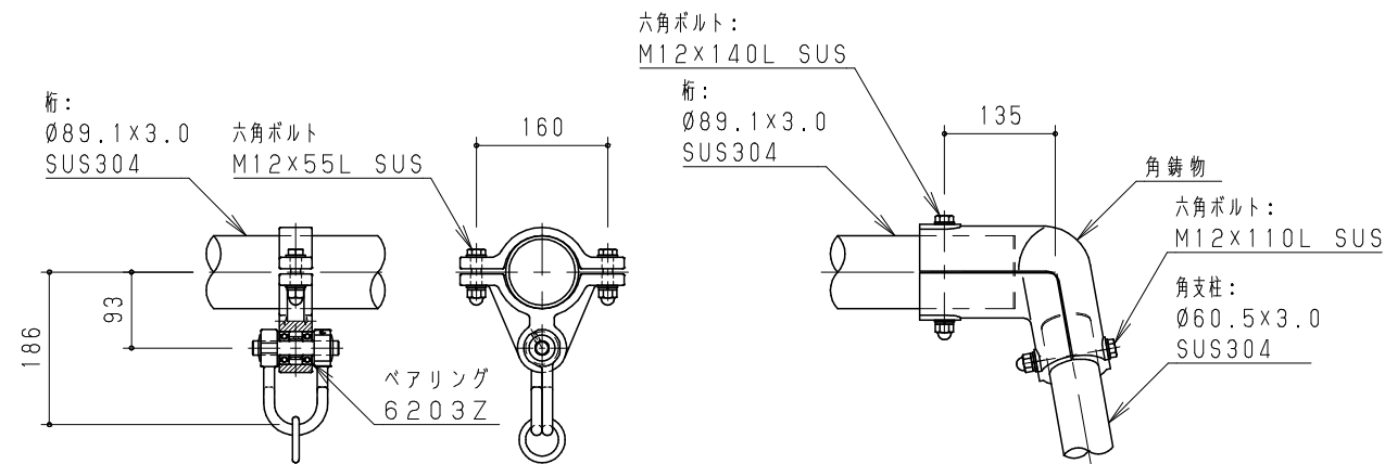
クラッチ詳細図 S = 1 / 10
