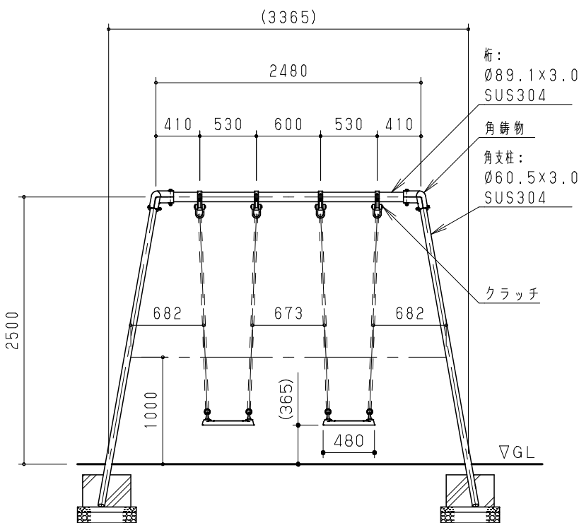
立面図 S = 1 / 50
