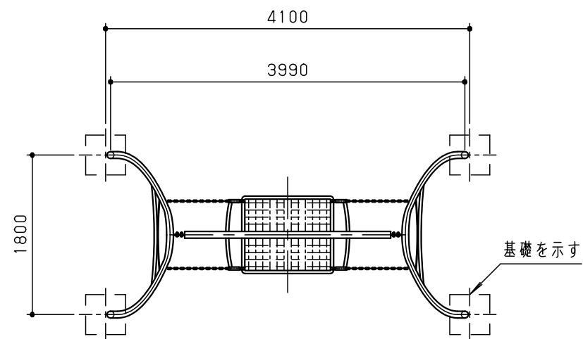
平面図 S = 1 / 60
