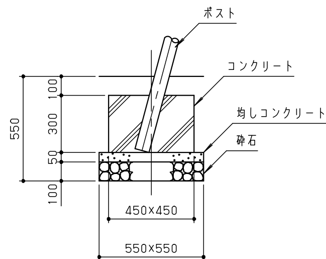
プランコ基礎 S = 1 / 20
