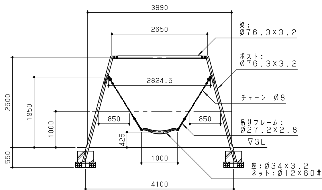
立面図 S = 1 / 60
