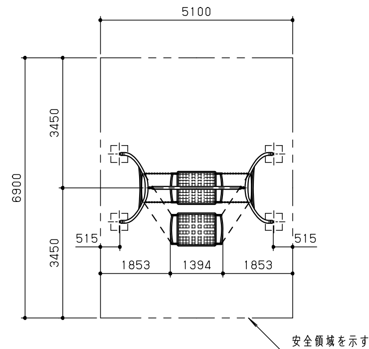
安全領域 S = 1 / 100
