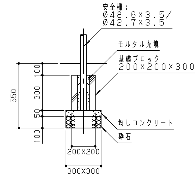
基礎断面詳細図 S = 1 / 20
