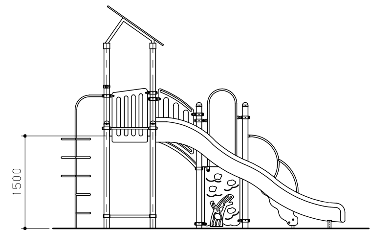
D 視立面図 S = 1 / 60
