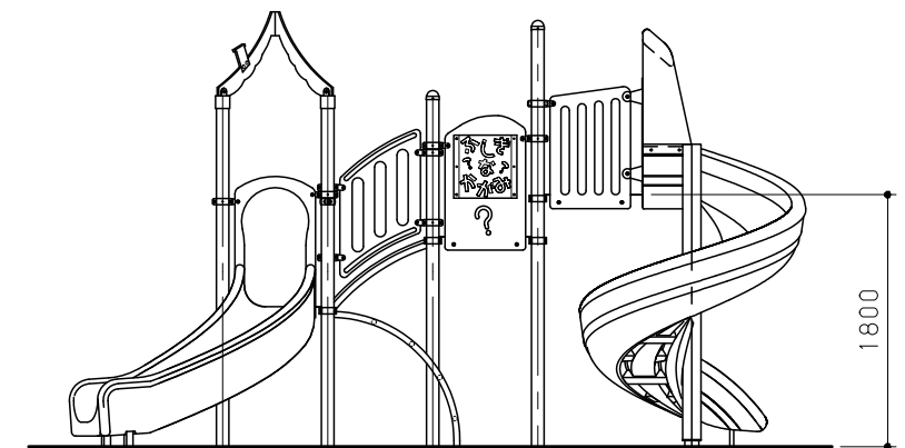
B 視立面図 S = 1 / 60
