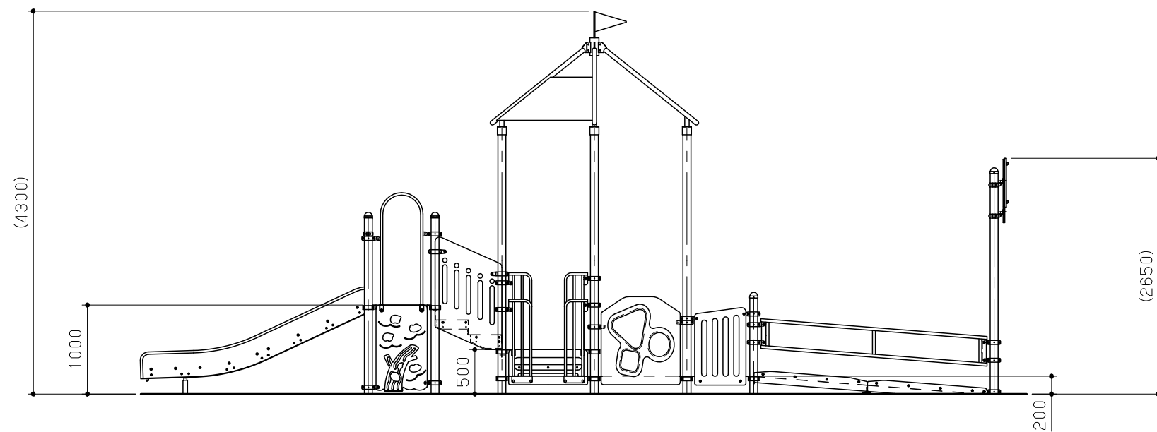
A 視立面図 S = 1 / 60
