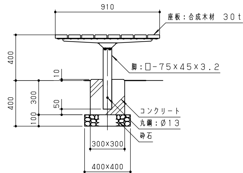
側面図 S = 1 / 20
