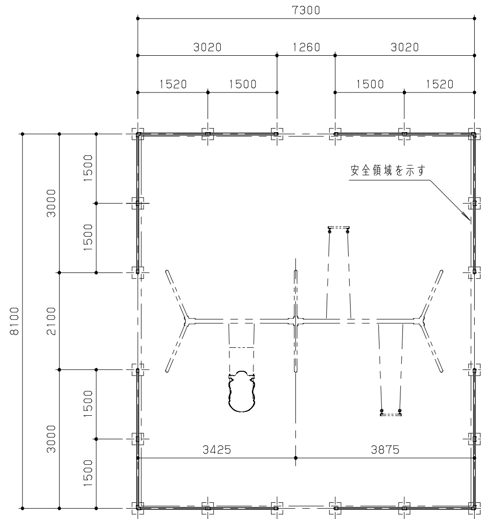
平面図 S = 1 / 80
