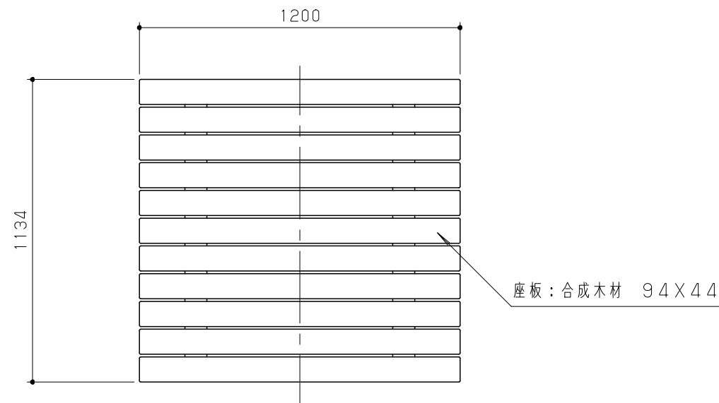
平面図 S = 1 / 20
