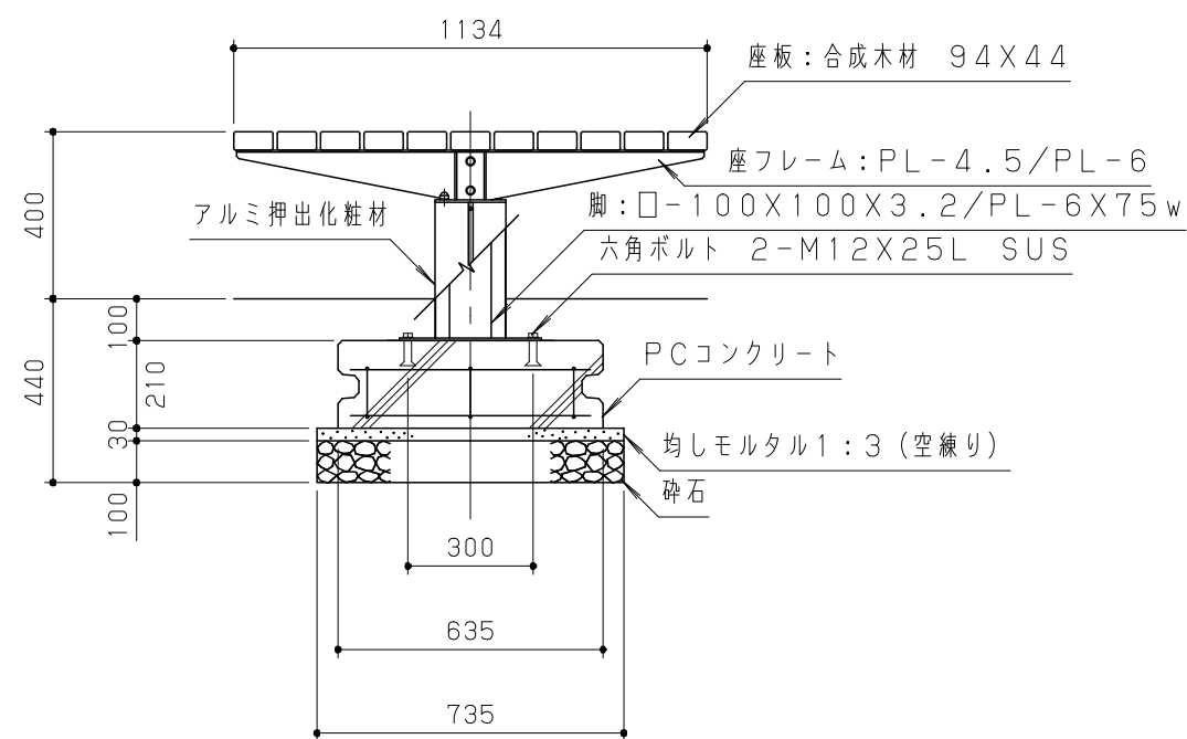
側面図 S = 1 / 20
