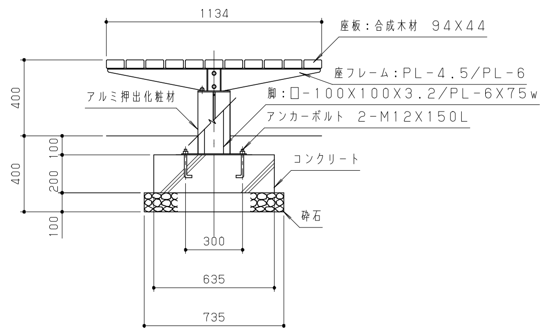
側面図 S = 1 / 20
