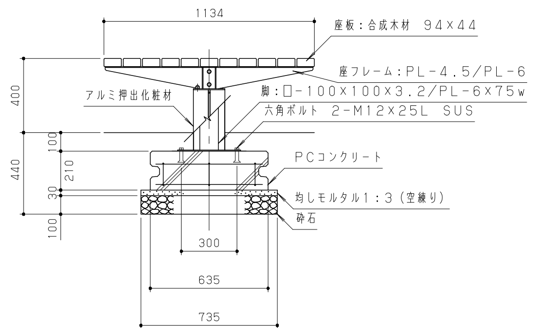
側面図 S = 1 / 20
