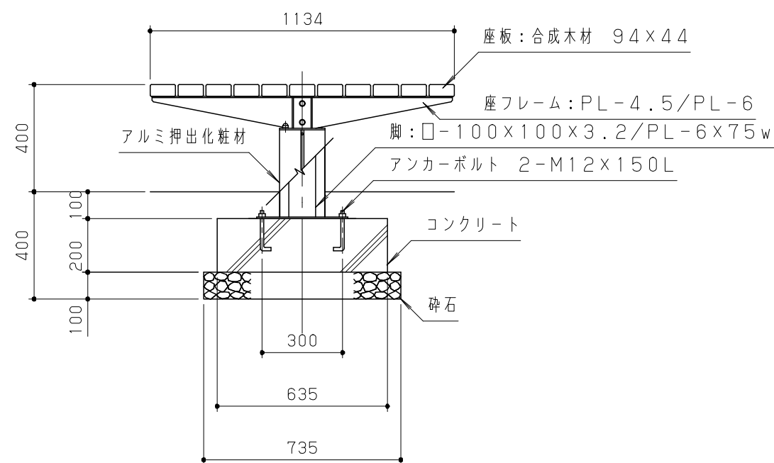
側面図 S = 1 / 20
