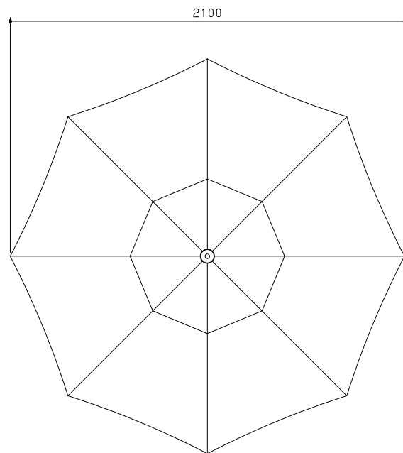
平面図 S = 1 / 20
