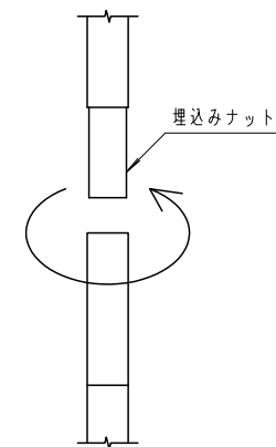
ジョイント詳細図 S = 1 / 5
