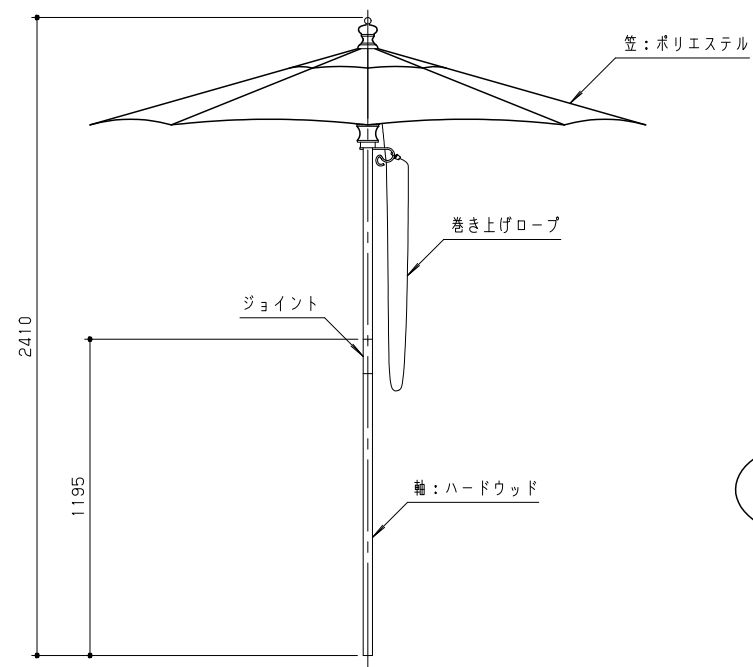
立面図 S = 1 / 20
