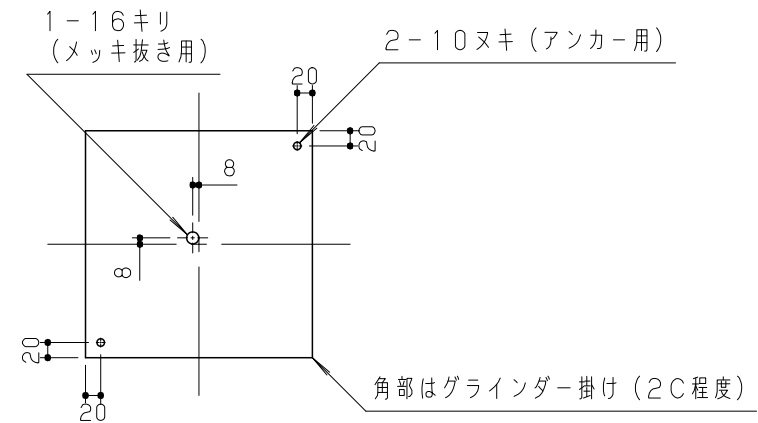
ベース加工図 S = 1 / 10
