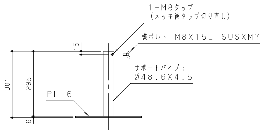
立面図 S = 1 / 10
