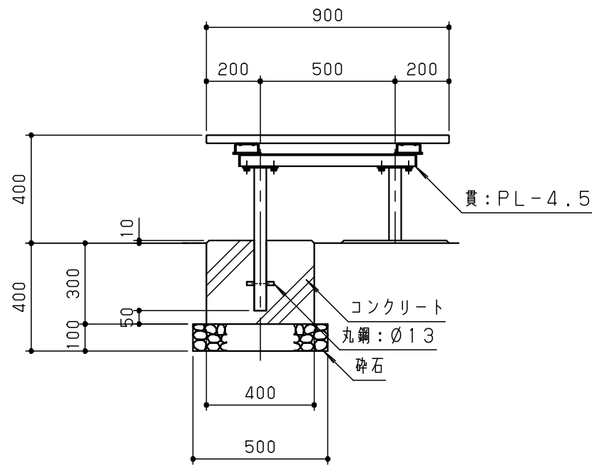
立面図 S = 1 / 20
