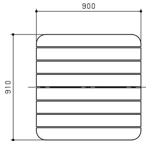
平面図 S = 1 / 20
