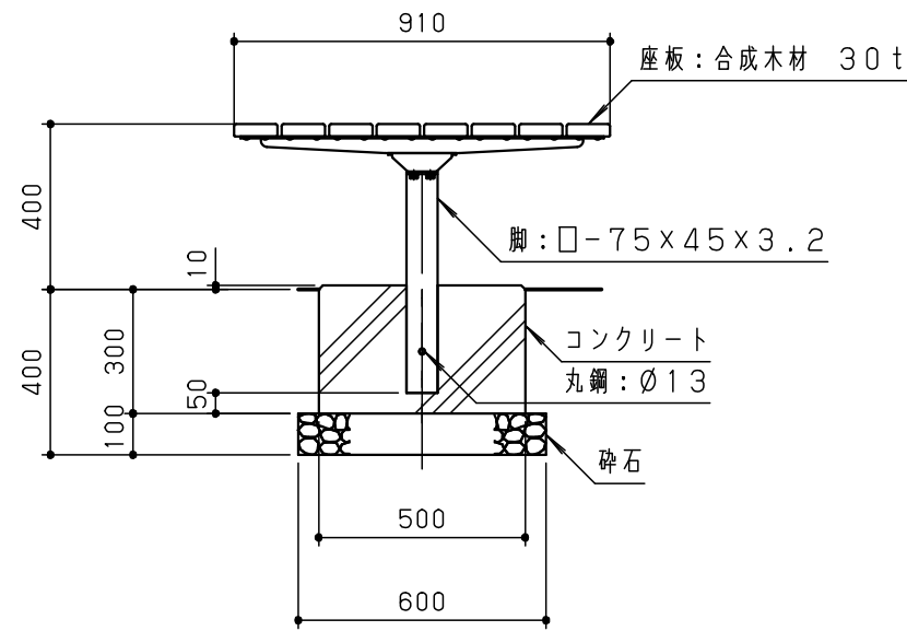
側面図 S = 1 / 20
