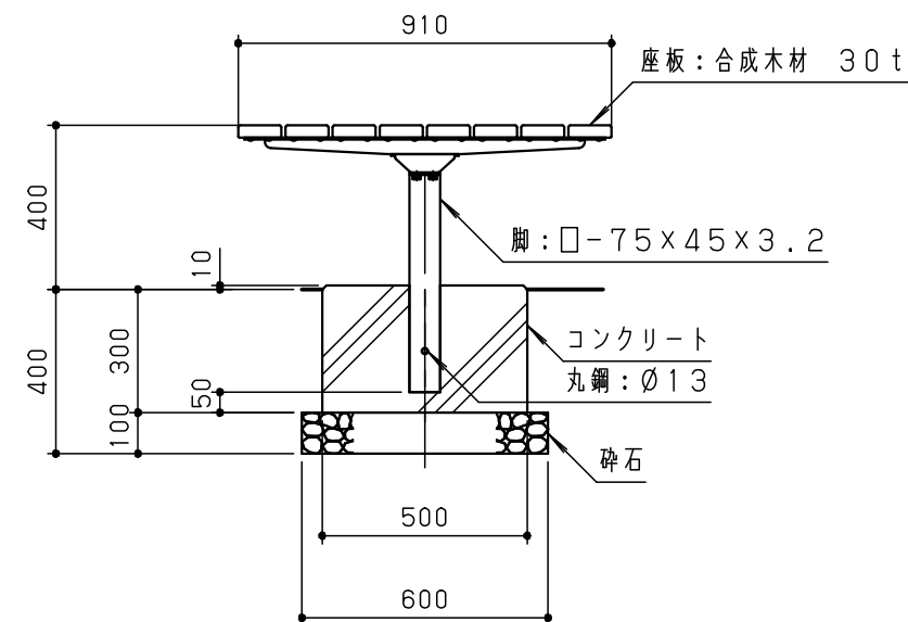
側面図 S = 1 / 20
