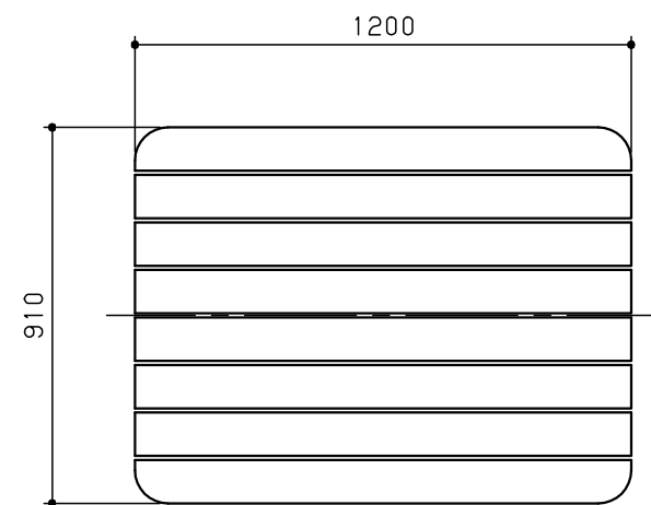
平面図 S = 1 / 20
