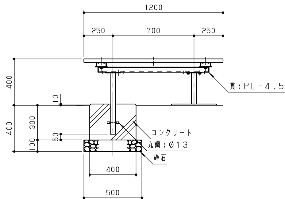
立面図 S = 1 / 20
