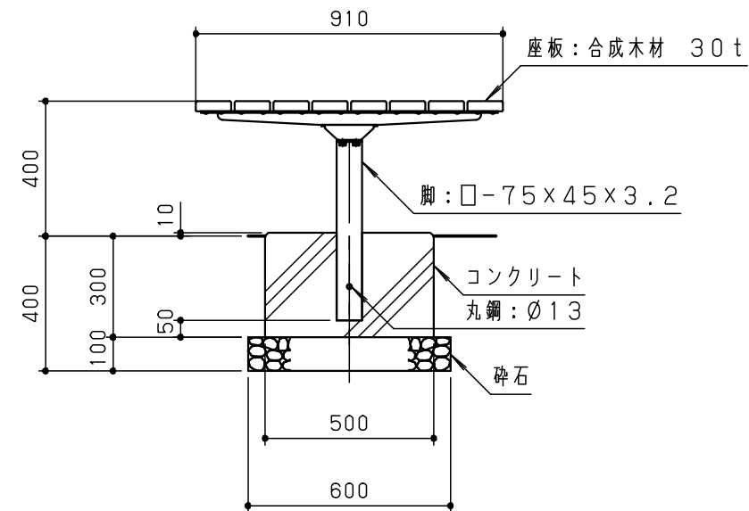
側面図 S = 1 / 20
