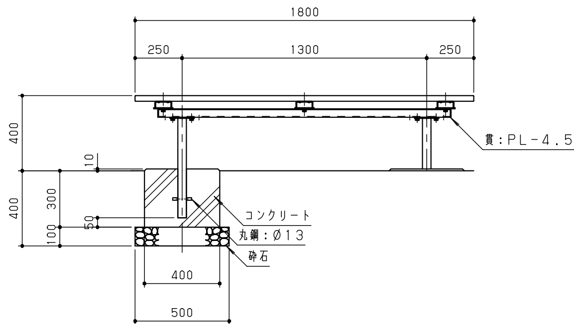
立面図 S = 1 / 20
