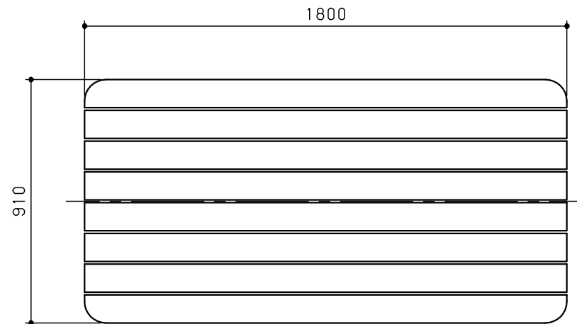
平面図 S = 1 / 20
