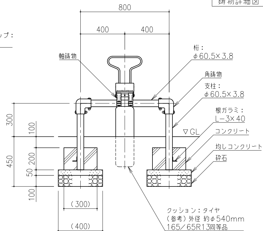
鑄物詳細図 S=1/10
