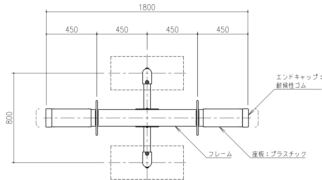
平面図 S=1/20
